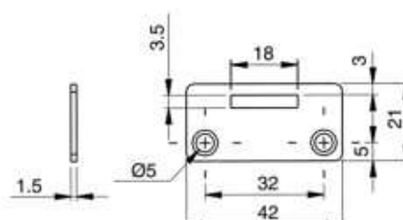
Alulra szerelt zár kétszárnyú ajtóra
