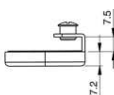
Felülre szerelt zár egyszárnyú ajtóra
