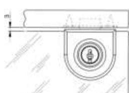
Felülre szerelt zár egyszárnyú ajtóra
