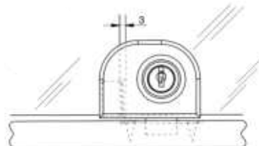
Alulra szerelt zár kétszárnyú ajtóra
